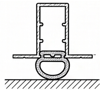
Extendido Sello Desplegado Contra el Suelo
