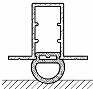
Reposo Sello Retraido
