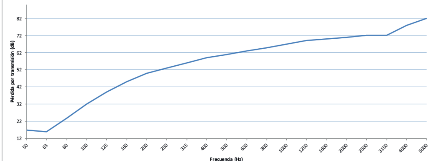
Pérdida por transmisión de la partición (Transmission Loss)
